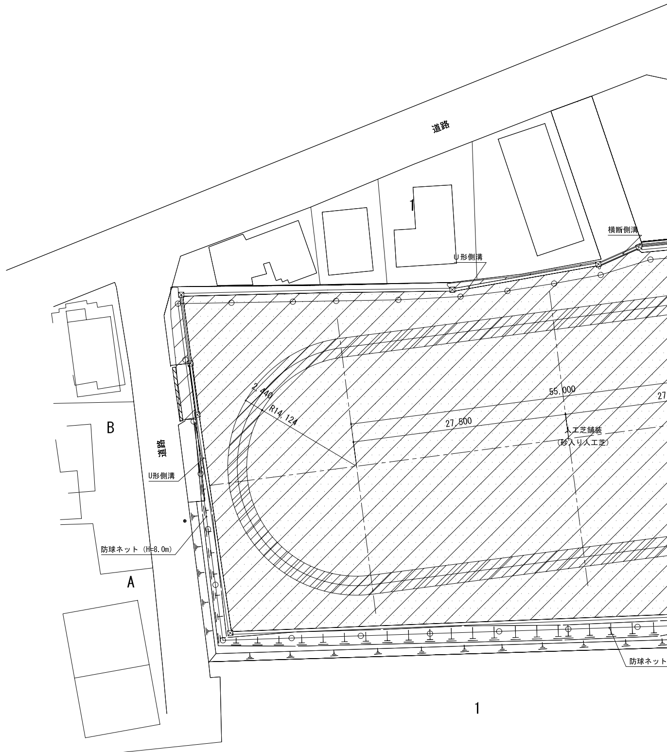
計画平面図 ⑤
